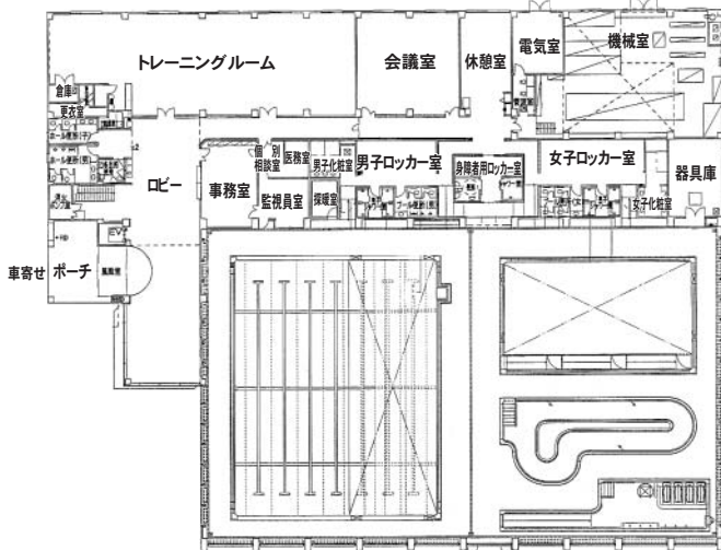
1階キープラン
